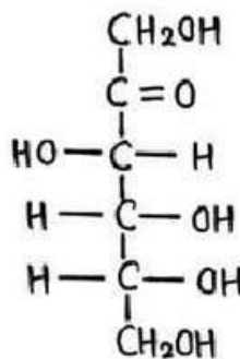
Ketoses
