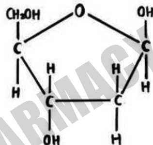
DEOXYRIBOSE
