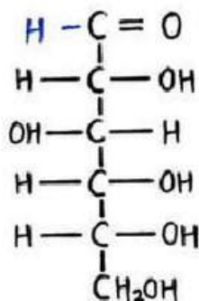
Aldoses
