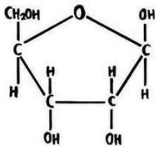
RIBOSE
