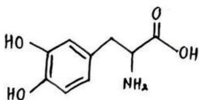
L- Dopa
