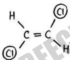
trans - 1,2 - dichloroethane
