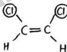
cis - 1,2, dichloroethane
