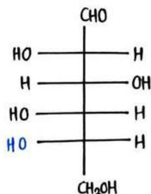
L- Glucose
