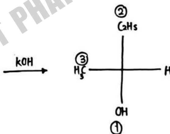
③ - 2-Butanol
